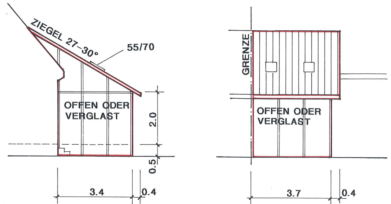
MST. 1 : 100
