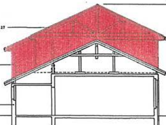
SCHNITT A-A 1:100
